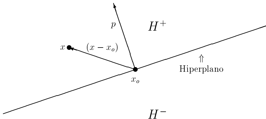
Figura 2.6: Subespacios
