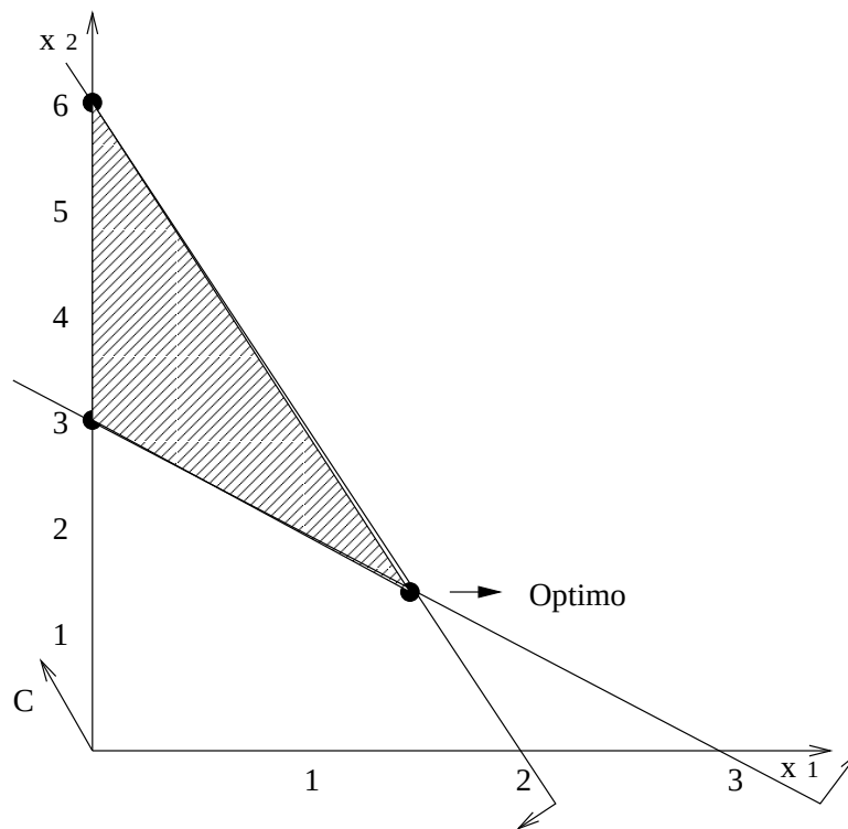
Figura 7.1: Problema primal.
